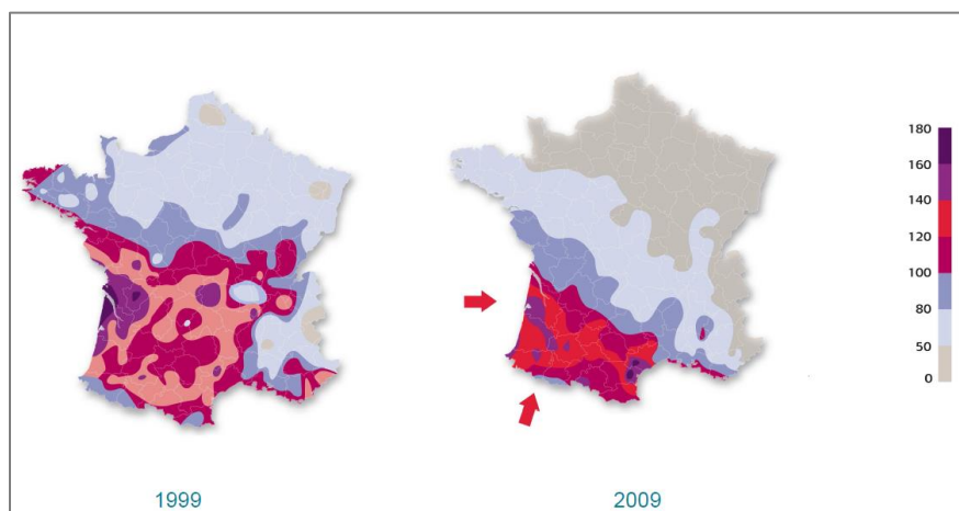
Figure 41 Vitesses instantanées des vents de tempêtes de 1999 et 2009. Bilan de la tempête Klaus, ERDF, 2009
