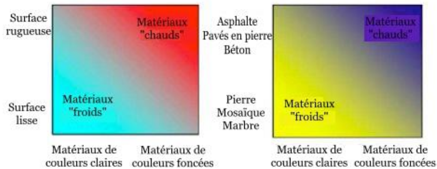
Figure 28 Matériaux « chauds » et matériaux « froids », Musy, 2007
