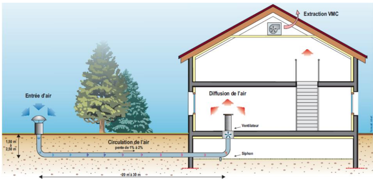
Figure 49 Schéma de principe d'un puits canadien. CETE de Lyon, 2005
