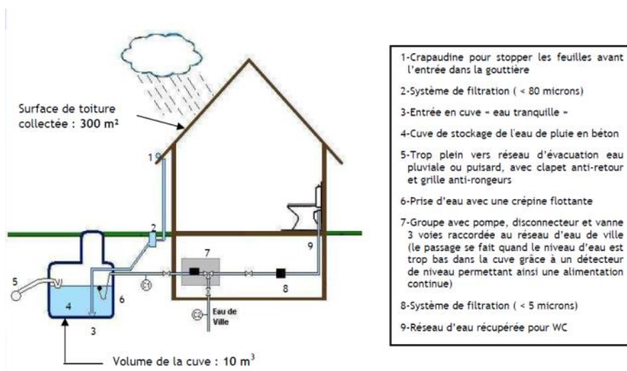
Figure 17 Schéma de principe d'un système de récupération de l'eau de pluie. Conseil Local à l'Énergie
