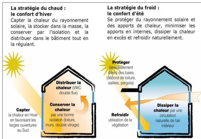
Figure 27 L'architecture bioclimatique, Traité d'architecture et d'urbanisme bioclimatique
