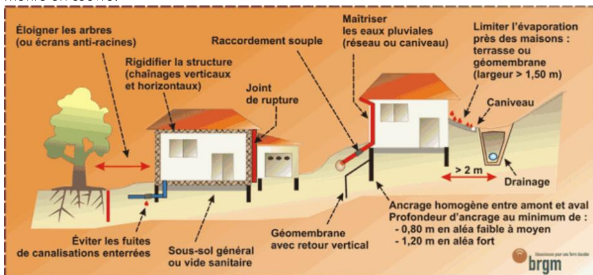
Figure 42 Les principes à mettre en œuvre pour construire sur terrain argileux. BRGM, 2010
