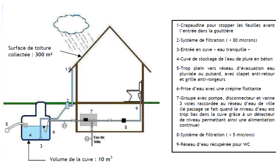
Figure 19 Schéma de principe d'un système de récupération de l'eau de pluie. Conseil Local à l'Energie
