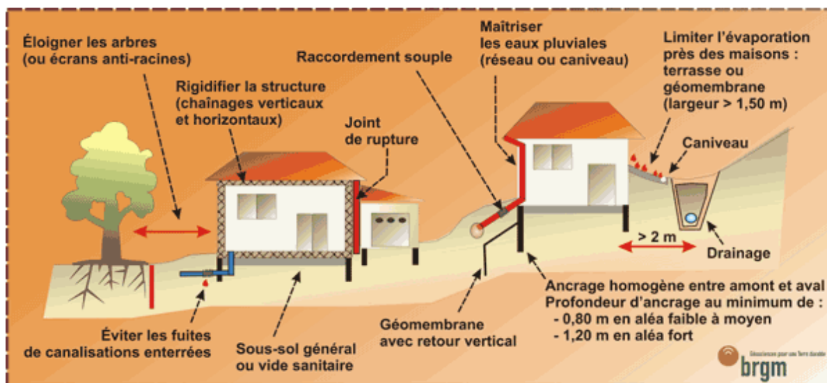
Figure 52 Les principes à mettre en œuvre pour construire sur terrain argileux. BRGM, 2010
