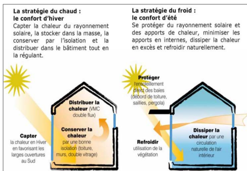
Figure 30 L'architecture bioclimatique, Traité d'architecture et d'urbanisme bioclimatique
