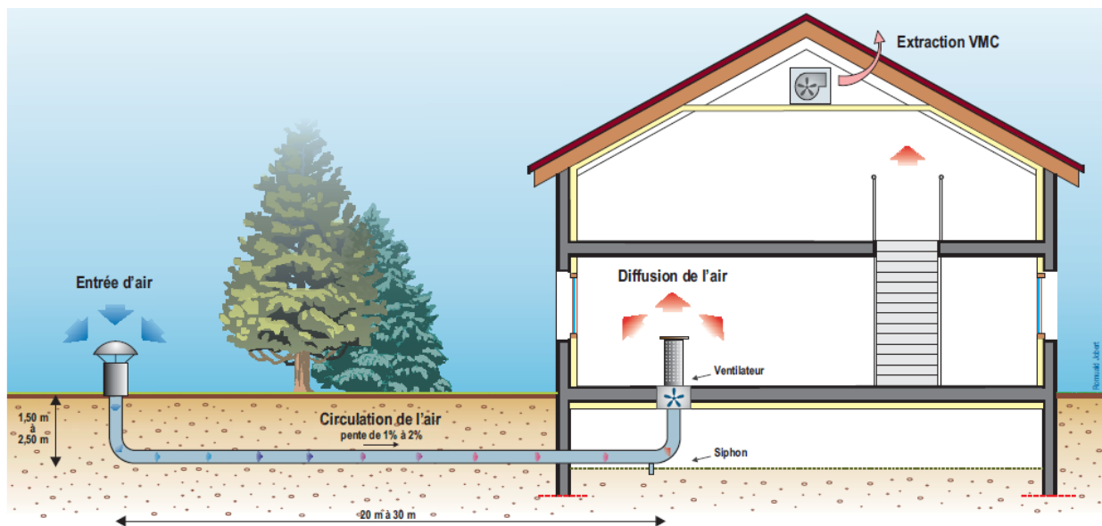
Figure 67 Schéma de principe d'un puits canadien. CETE de Lyon, 2005
