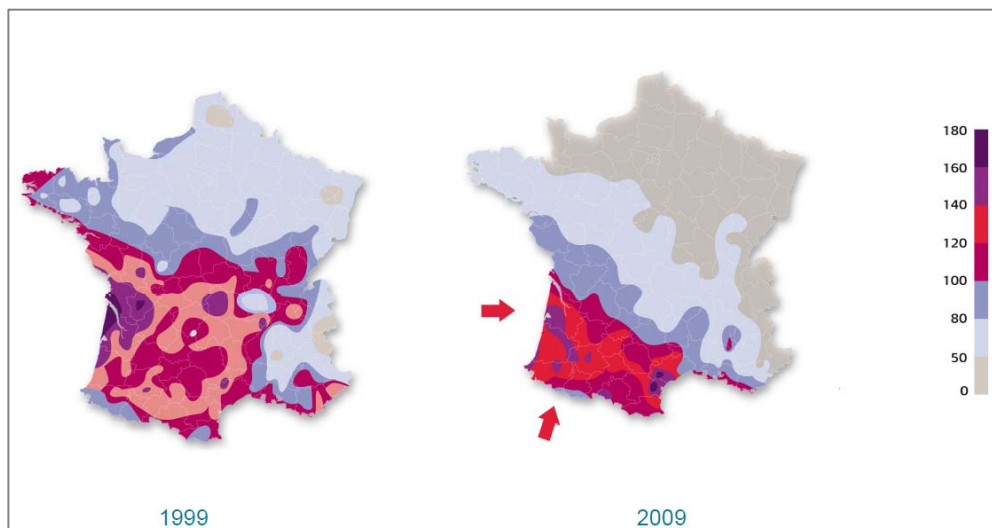
Figure 50 Vitesses instantanées des vents de tempêtes de 1999 et 2009. Bilan de la tempête Klaus, ERDF, 2009
