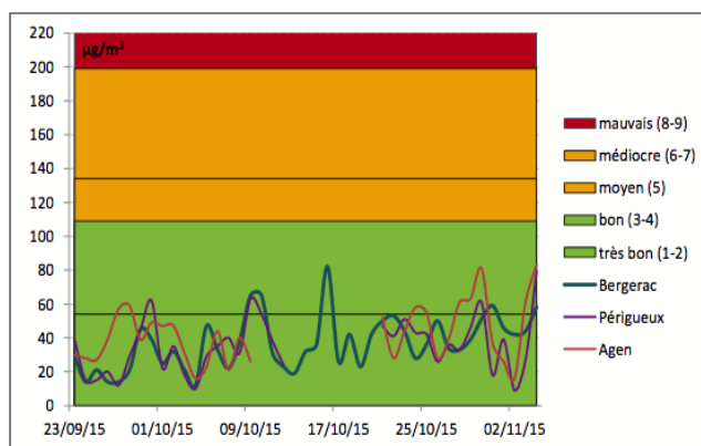
Figure 38 Evolution des maxima horaires en NO2. Evaluation de la qualité de l'air sur Bergerac, AIRAQ, 2015
