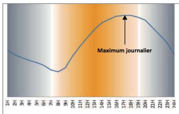
Figure 34 Profil typique de l'ozone au cours d'une journée. Evaluation de la qualité de l'air sur Bergerac, AIRAQ, 2015
