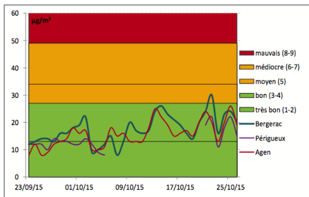
Figure 36 Evolution des moyennes journalières en PM10. Evaluation de la qualité de l'air sur Bergerac, AIRAQ, 2015
