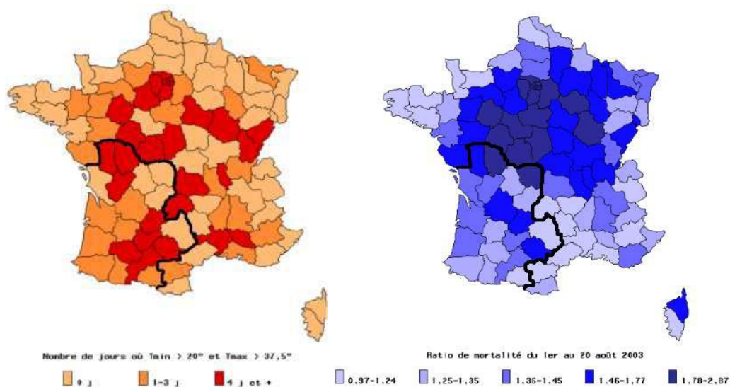
Figure 27 Nombre de jours de très fortes chaleurs au 1er au 20 août 2003 (à gauche) et ratio de surmortalité observé (à droite). INSERM, 2004
