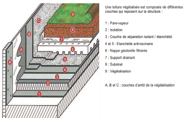
Figure 18 Schéma de principe d'une toiture végétalisée. Agence Locale de l'Energie de l'Agglomération Lyonnaise, 2008
