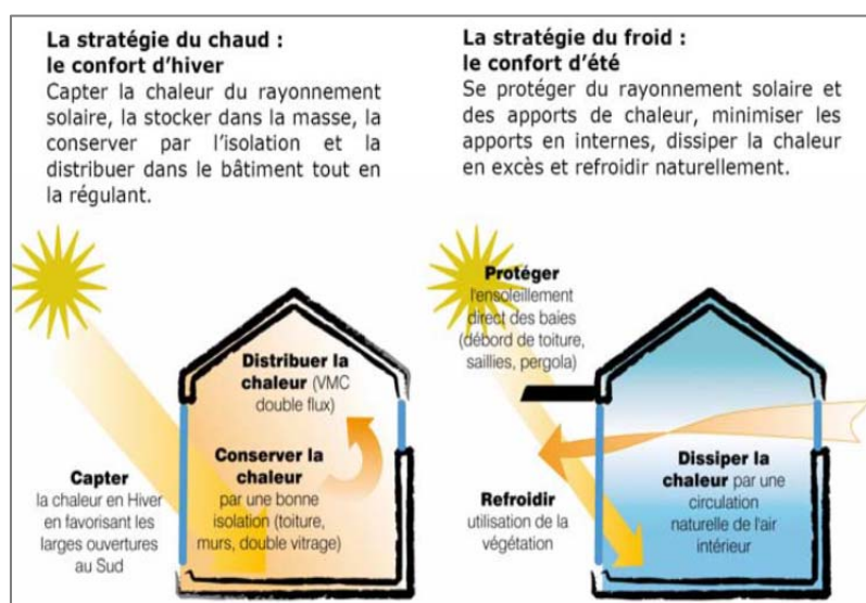
Figure 22 L'architecture bioclimatique, Traité d'architecture et d'urbanisme bioclimatique
