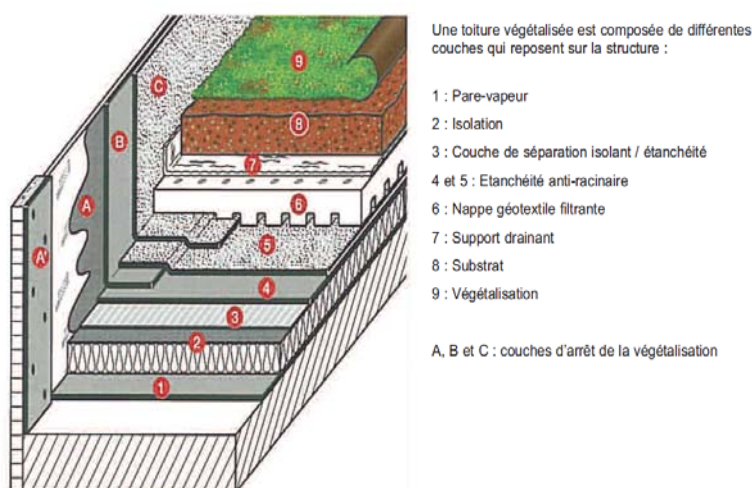
Figure 17 Schéma de principe d'une toiture végétalisée. Agence Locale de l'Energie de l'Agglomération Lyonnaise, 2008
