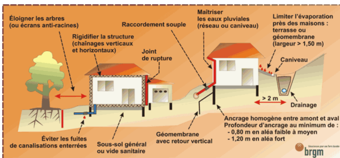
Figure 31 Les principes à mettre en œuvre pour construire sur terrain argileux. BRGM, 2010
