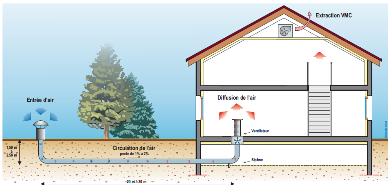
Figure 37 Schéma de principe d'un puits canadien. CETE de Lyon, 2005
